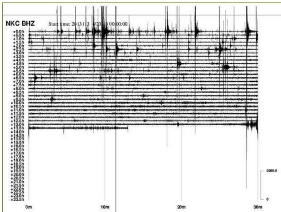
Záznam z posledního zaznamenaného zemětřesení na Kraslicku dne 23. 4. 2013.
