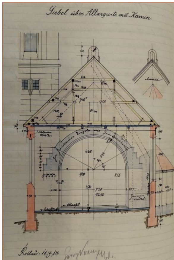
Část výkresu projektu kostela od A. Möllera.
