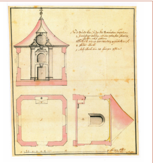
Obr .3: Žitná (okr. Sokolov), plán zámecké kaple z ledna 1756, zobrazující nárys části vstupního průčelí kaple s příčným řezem jejími bočními zdmi, plán přízemí a podélný řez kaplí mezi vstupem a oltářem. Originál v majetku Arcibiskupství pražského, uložen v Národním archivu.
