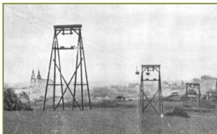
Visutá lanová dráha pro dopravu uhlí z dolu Arnošt-Ludmila v Kynšperku do textilní továrny v Libavském Údolí.
