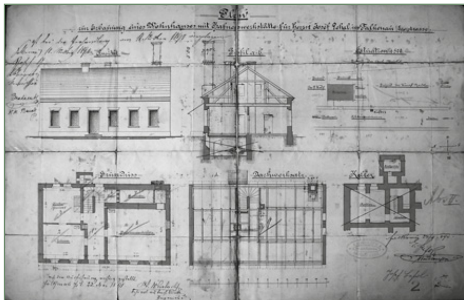
Dům s hrnčířskou dílnou v Chebské ulici z roku 1891 pro J. Pehala. Projektoval a stavěl stav. E. Lifka. Sklep nebyl povolen.
