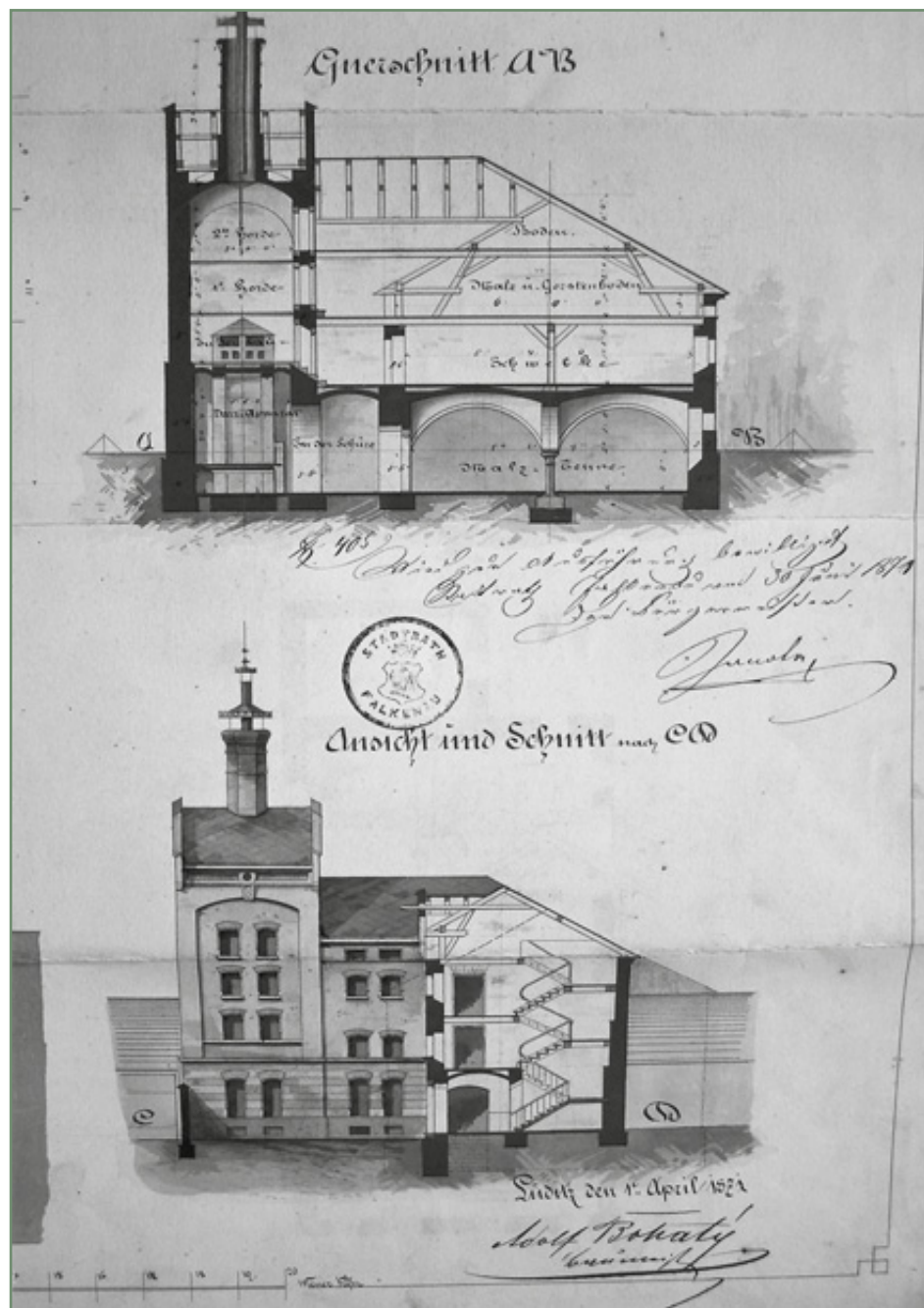
Projekt měšťanského pivovaru vypracovaný A. Bohatým ze Žlutic
