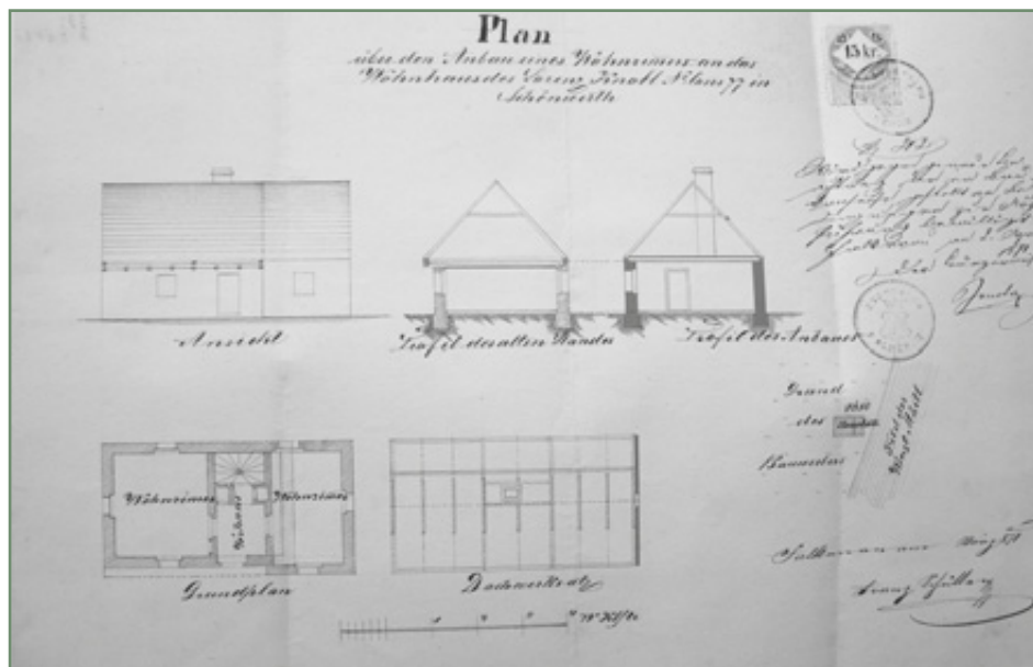
Plán přístavby čp. 77 na Šenverte, potvrzený v roce 1871 starostou Janotou a zednickým mistrem Franzem Schullanym.
