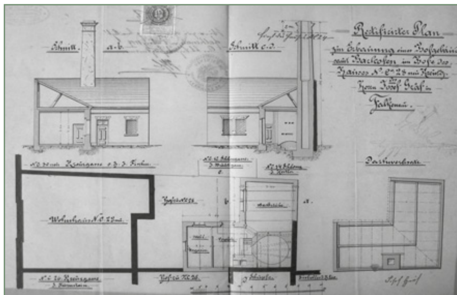
Příklad výkresu čp. 28 pro J. Grafa. Projektantem a stavelem byl E. Lifka. Projekt potvrdil tehdejší starosta Wenzl Fritsch v roce 1879.
