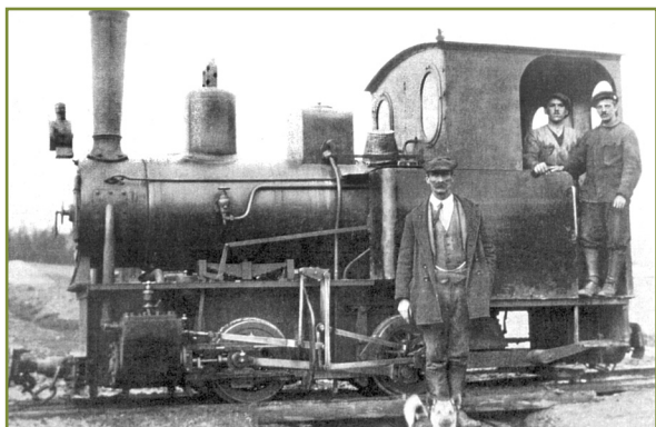
Na obrázku je dobře vidět jednoduchou konstrukci lokomotivy Orenstein & Koppel, typ Bt.
