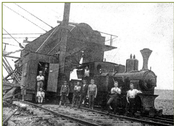
Lokomotiva s vozíky pod násypkou korečkového rypadla.
