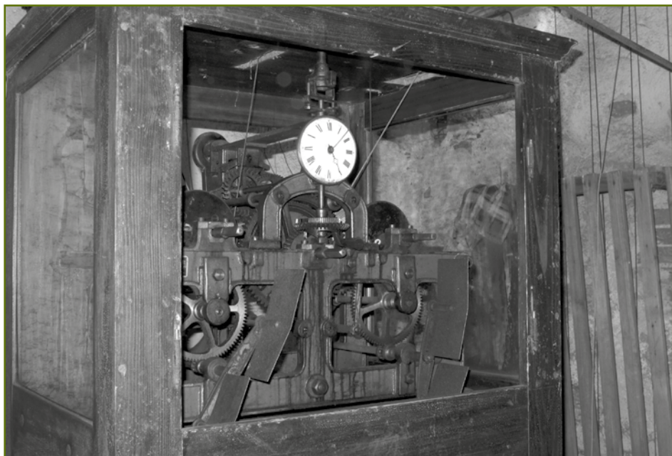
Hodinový stroj v kostele sv. Petra a Pavla v Krajkové před restaurováním. Foto L. Smola 2013.
