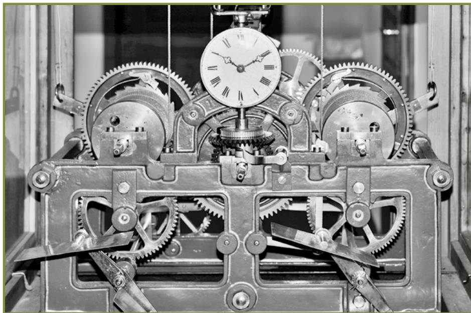
Hodinový stroj v muzeu v Horním Slavkově. Foto L. Smola 2015.
