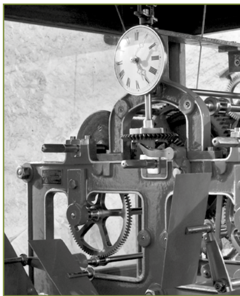
Hodinový stroj v kostele sv. Petra a Pavla v Krajkové po restaurování. Foto L. Smola 2014.
